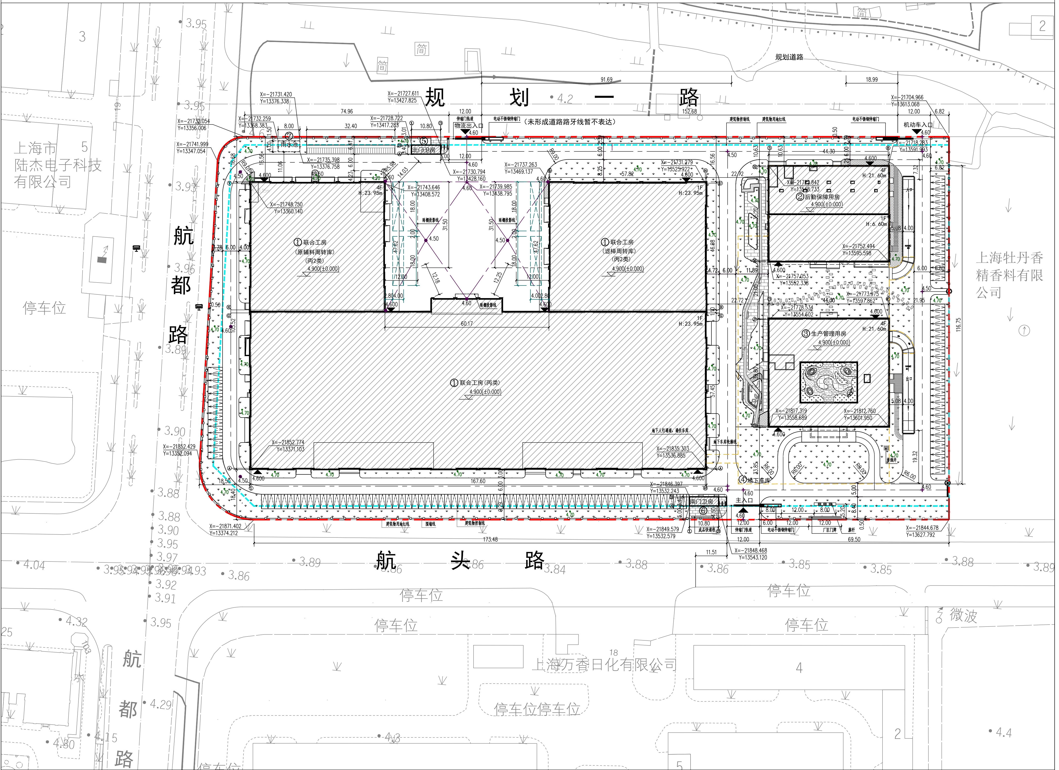
总平面图 1:750
