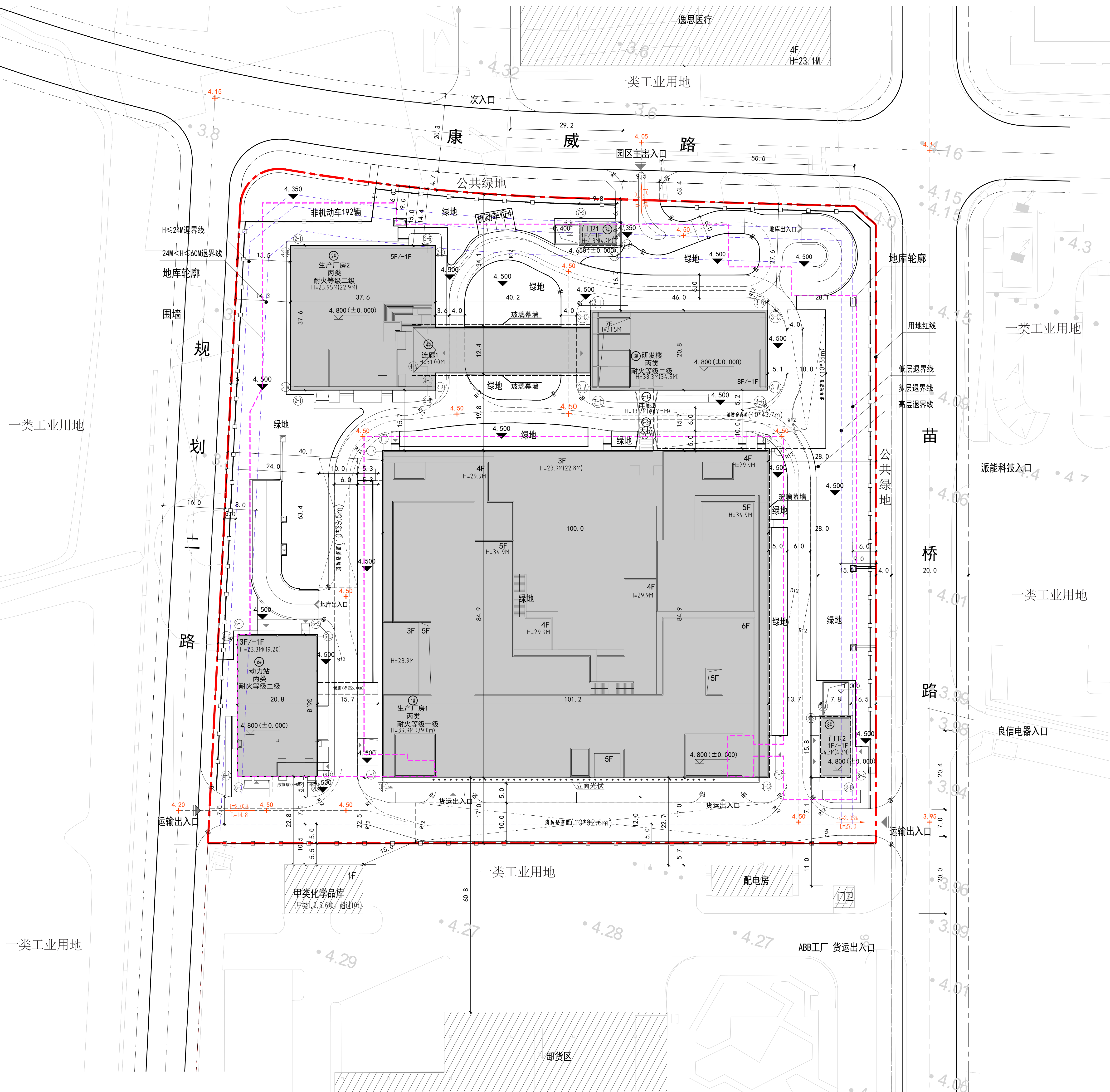
总平面图
