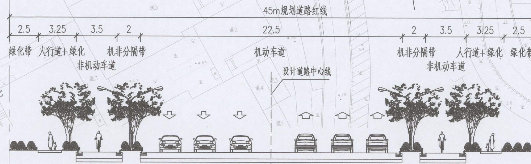
秀浦路标准横断面
