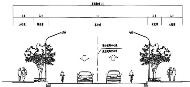
道路标准横断面
