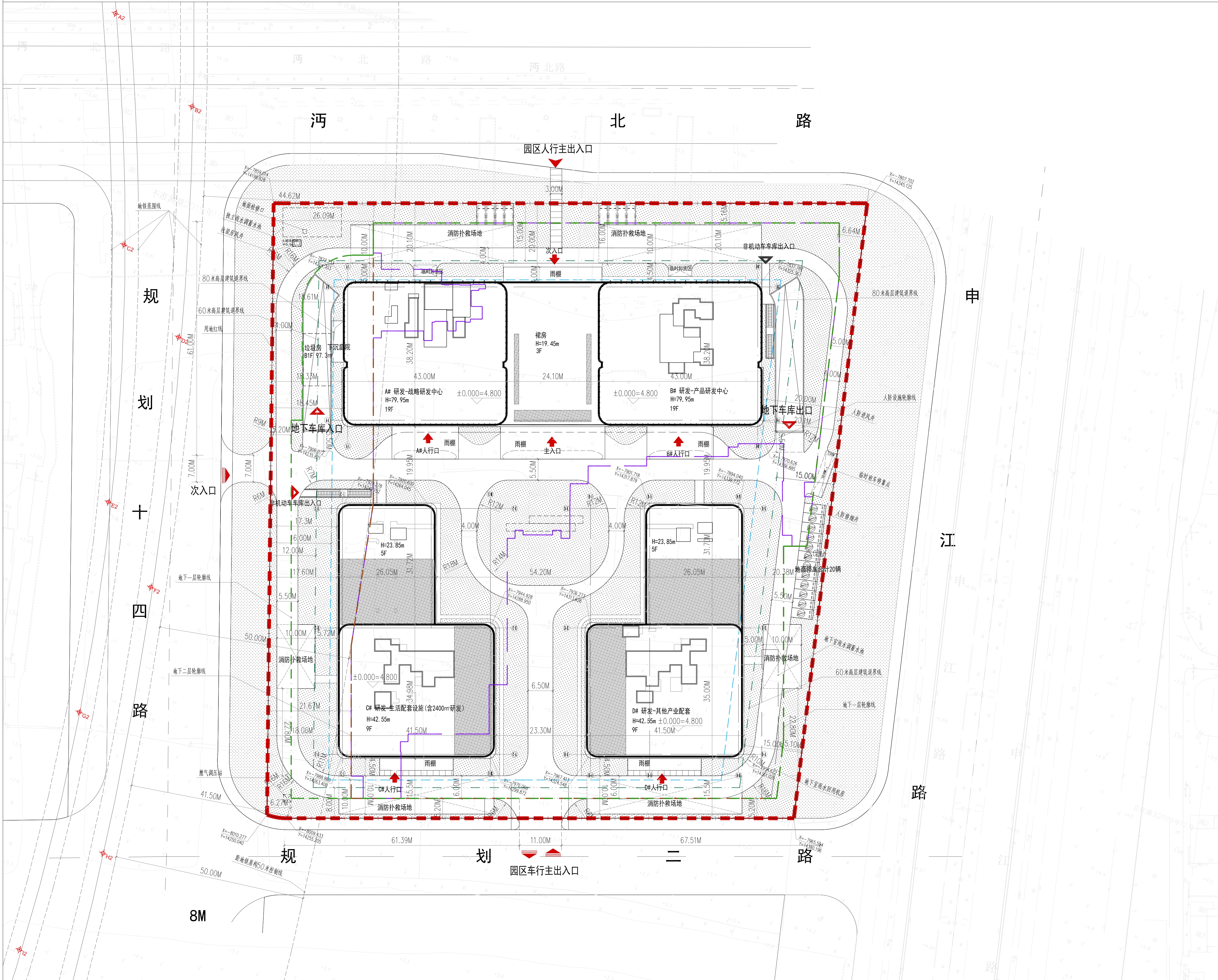
总平面图
