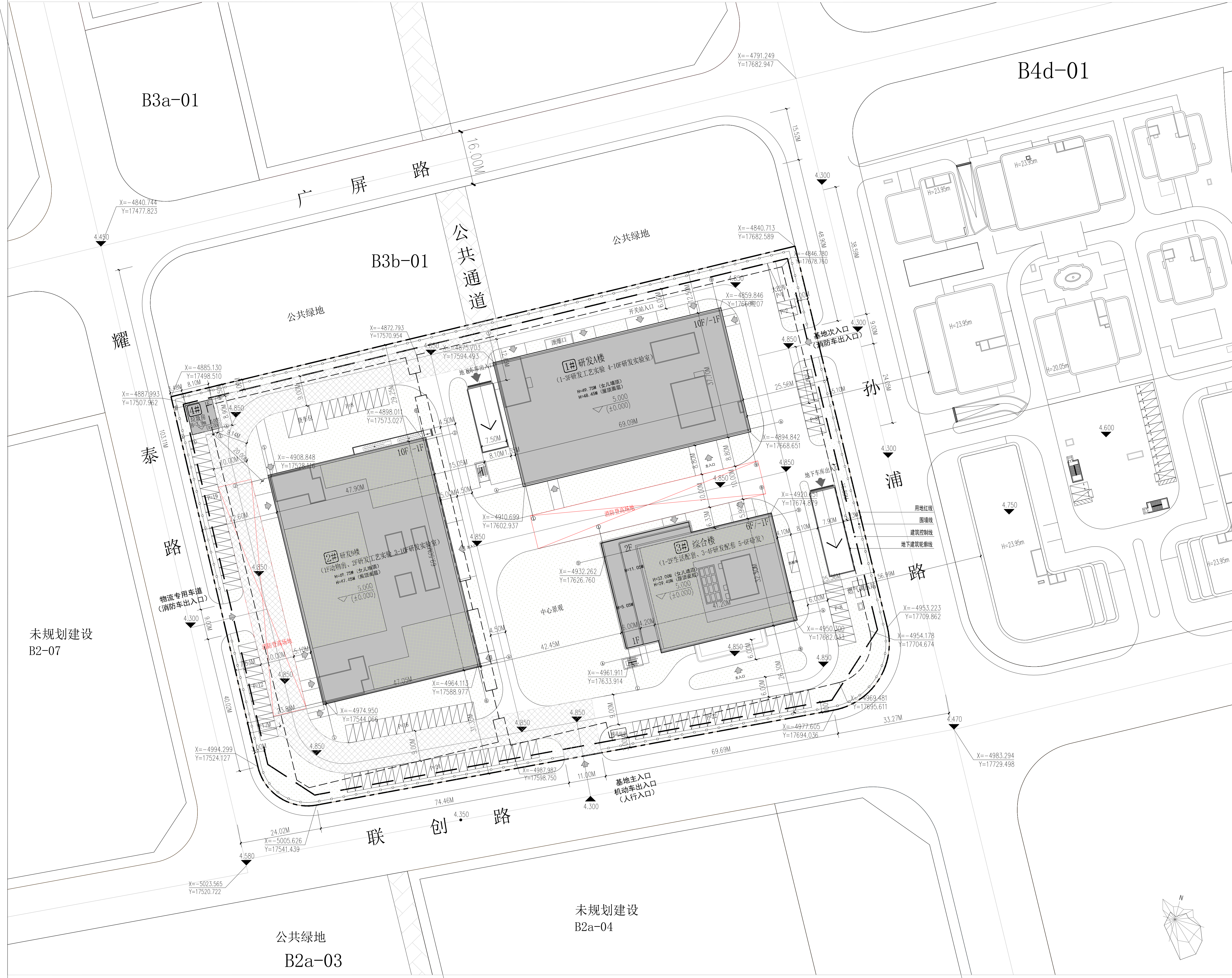
总平面图
