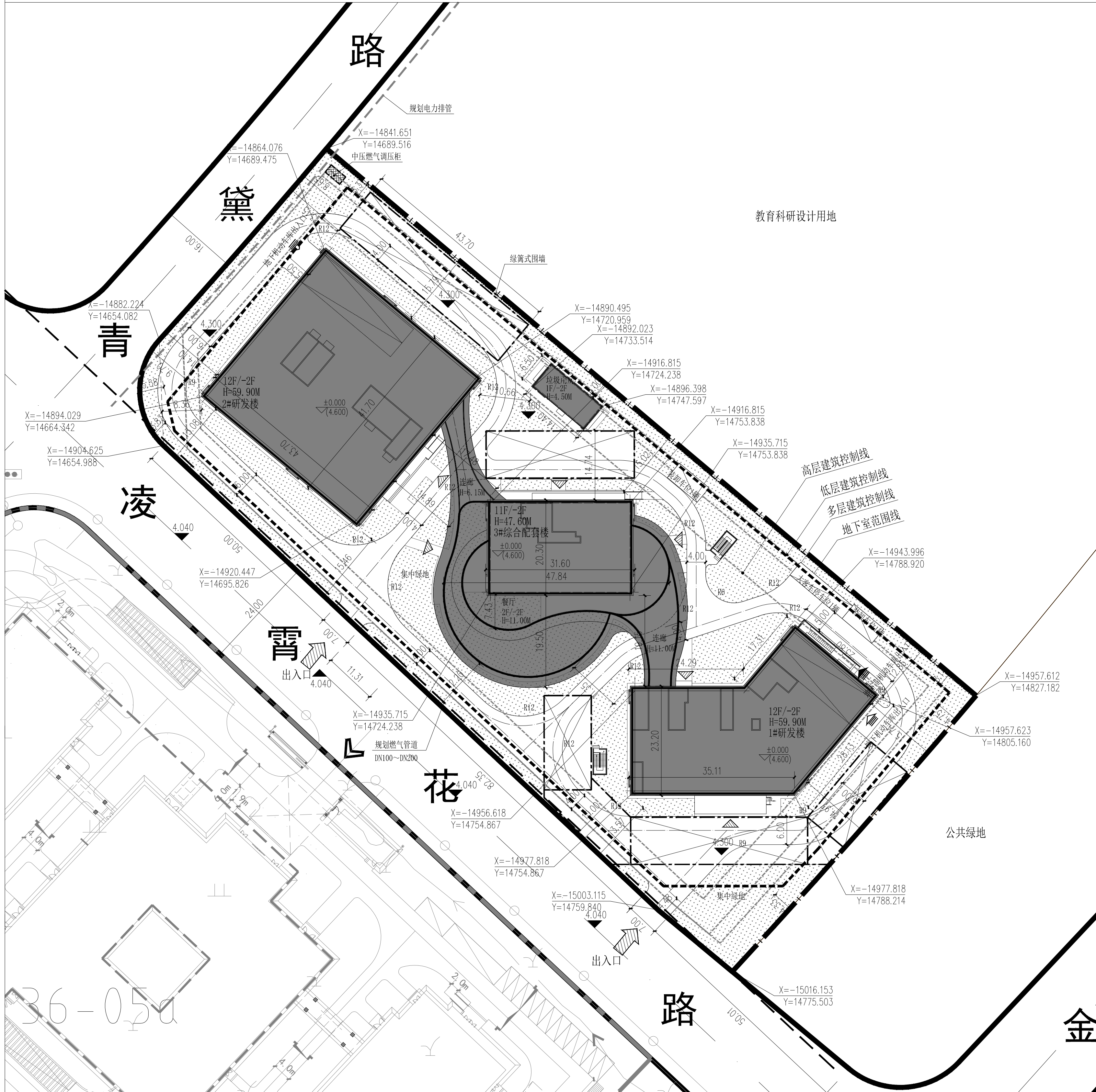
总平面图
